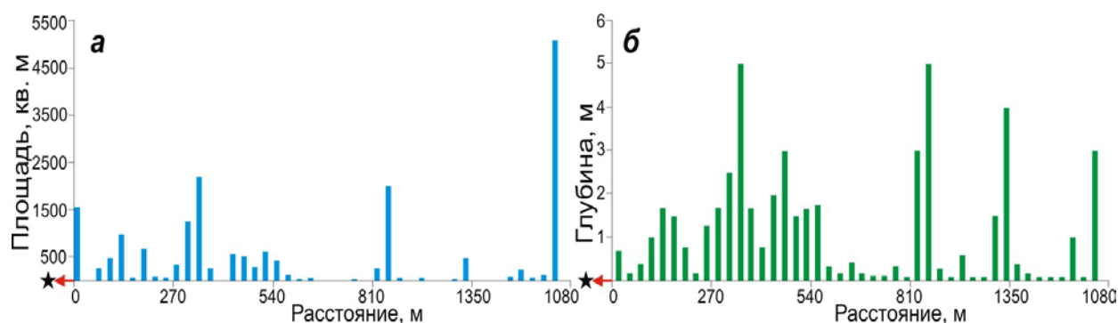
Рис. 5. Гистограммы распределения воронок-провалов на удалении от эпицентра Мондинского землетрясения 1950 г.: a — по максимальной площади ( \text{м}^2 ); б — по максимальной глубине (м).
